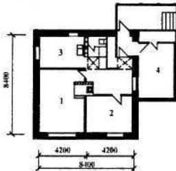
ПЛАН ЭТАЖА
