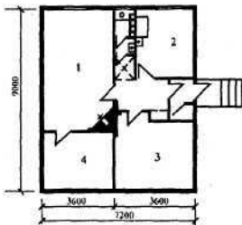
ПЛАН ЭТАЖА
