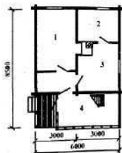
ПЛАН ПЕРВОГО ЭТАЖА
